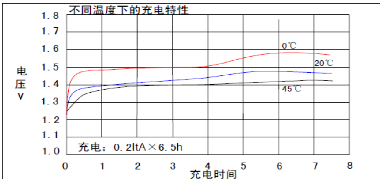
特征曲线
