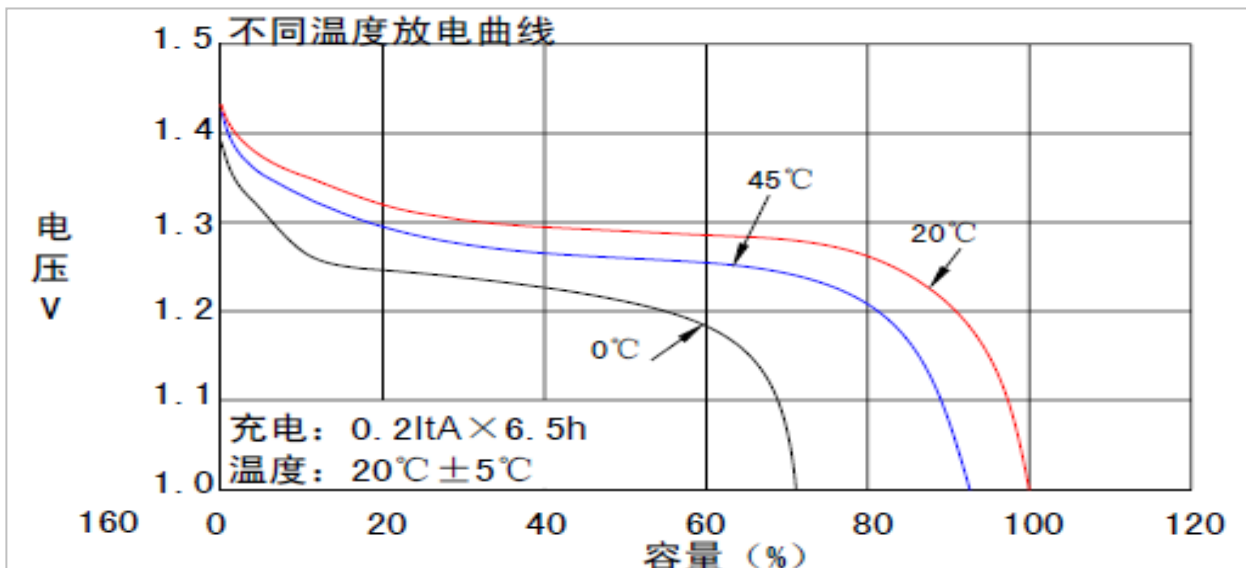
特征曲线
