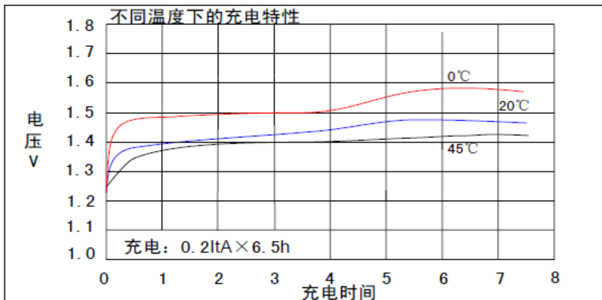
特征曲线
