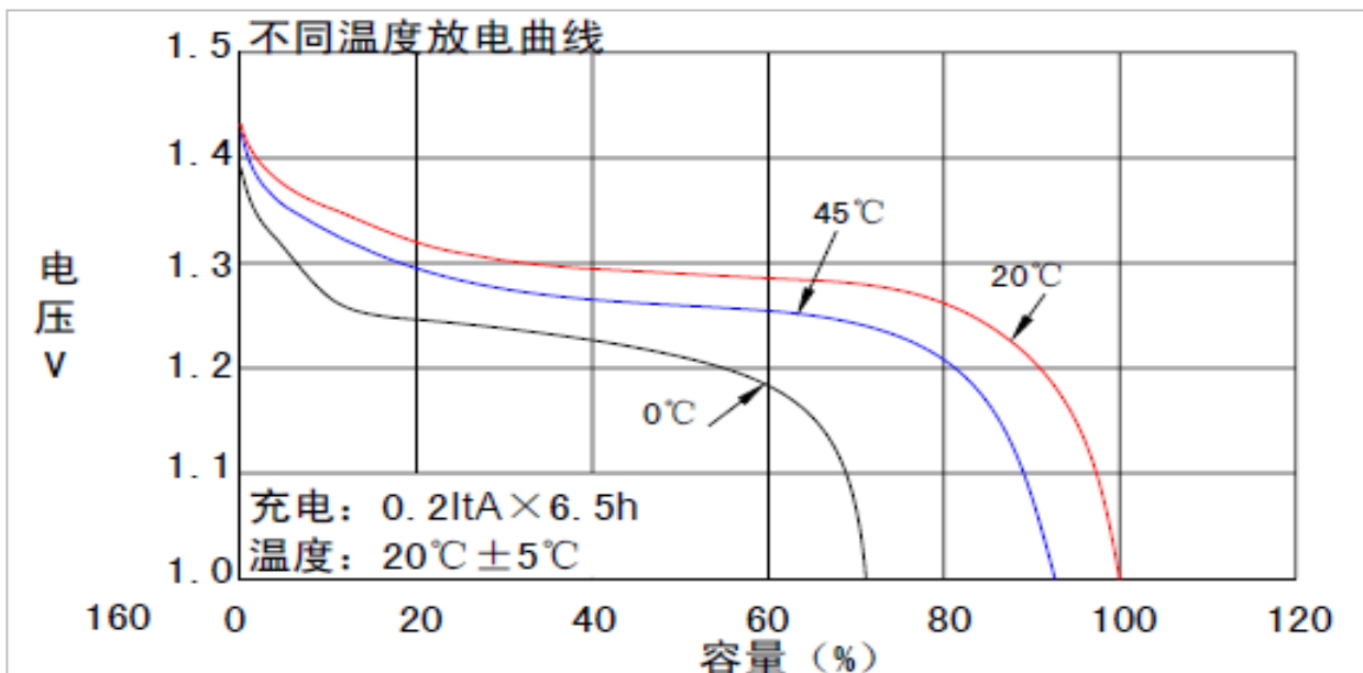
特征曲线
