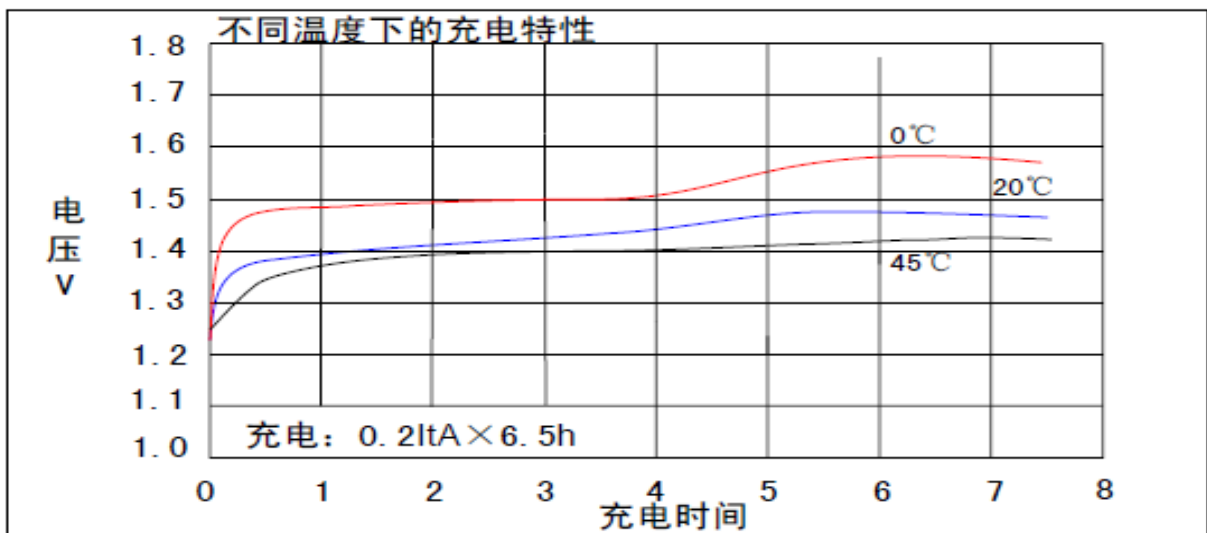
特征曲线
