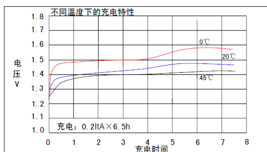
特征曲线
